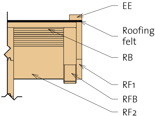
3 Facia
